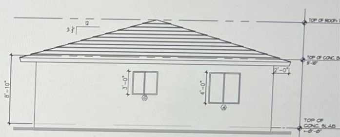
RIGHT ELEVATION SCALE: 1/4" = 1'-0"
